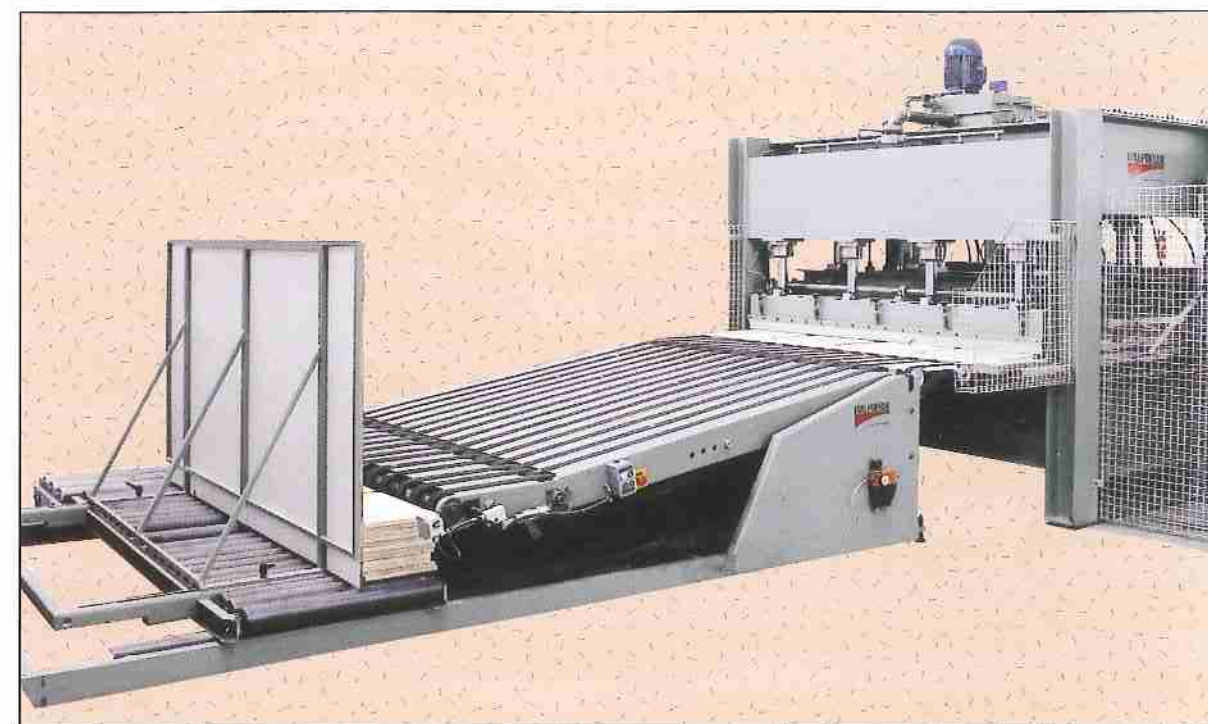
Détails des rouleaux de butée et de support groupe encollage.
